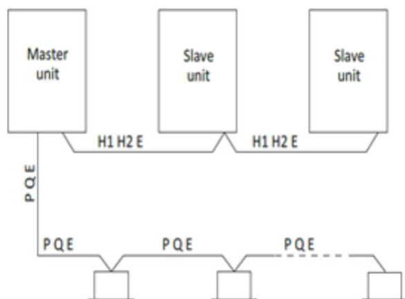
Connexion standard
